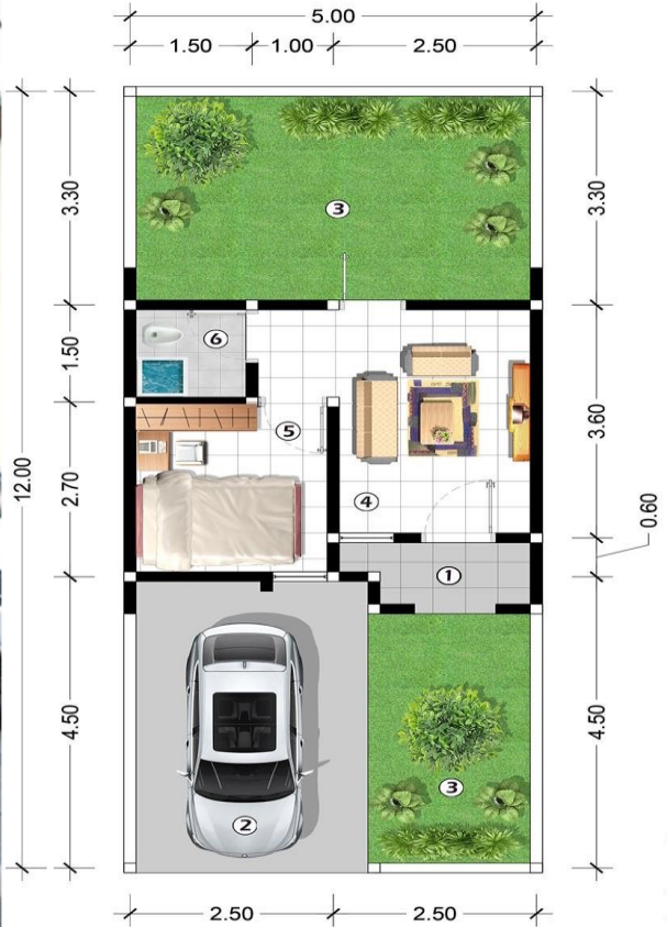
DENAH RUMAH TИPE 22/60 SKALA 1 : 50
